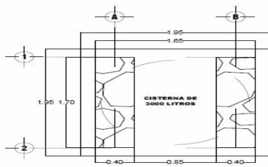
PLANTA ARQUITECTONICA
