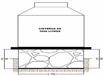
ALZADO LATERAL
